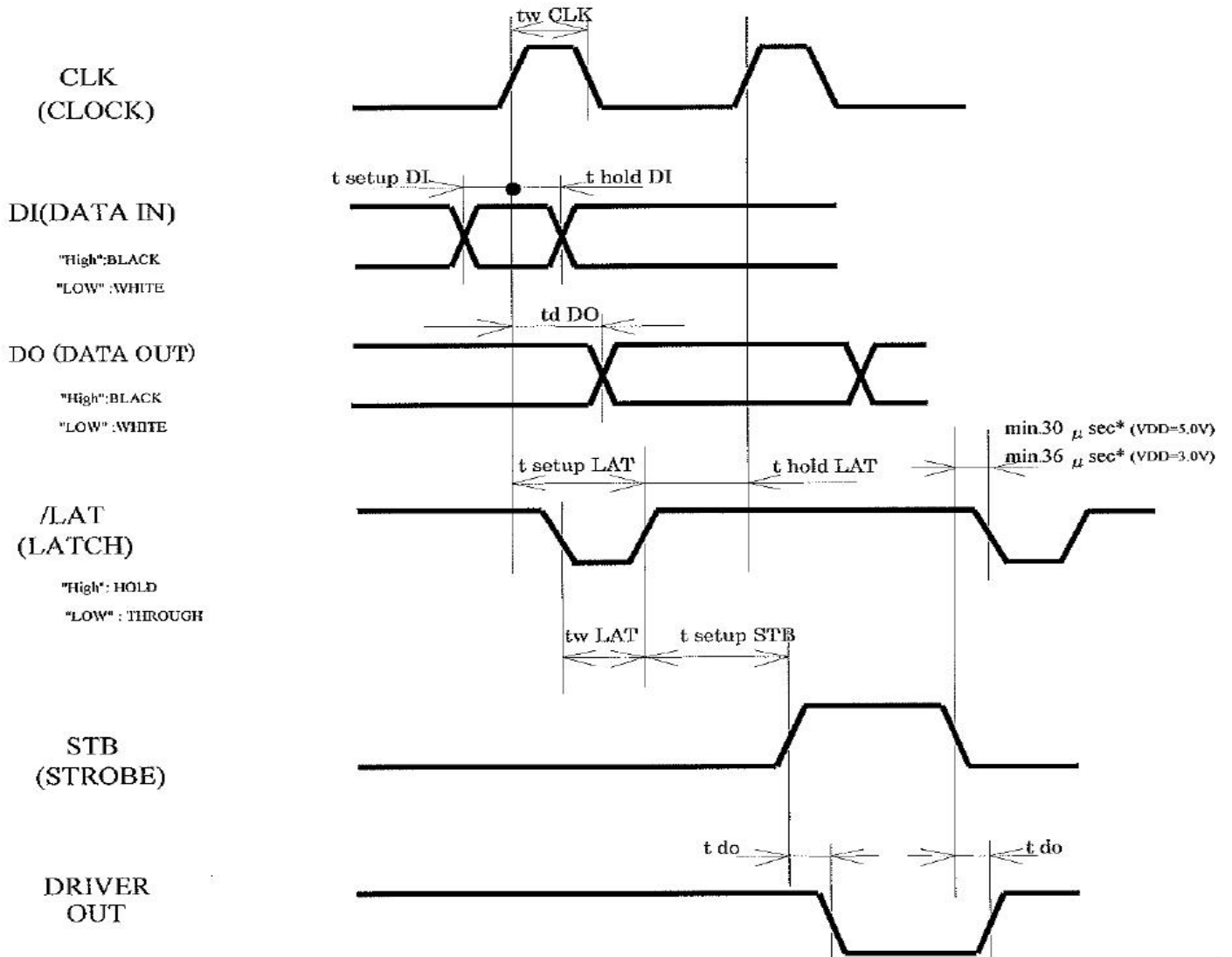
图 3 时序图
