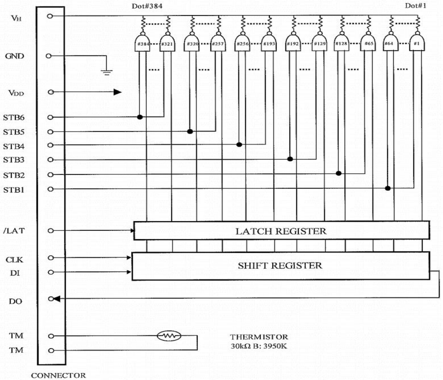
图 2 等价回路图
