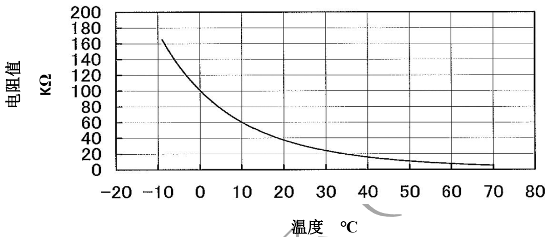
图 4 热敏电阻的温度特征
