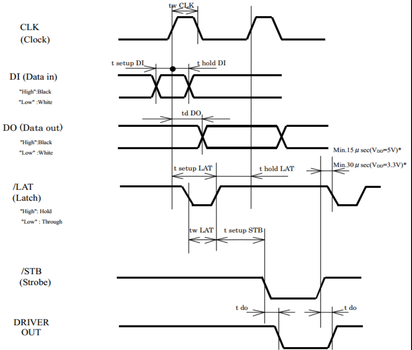
图 3 时序图
