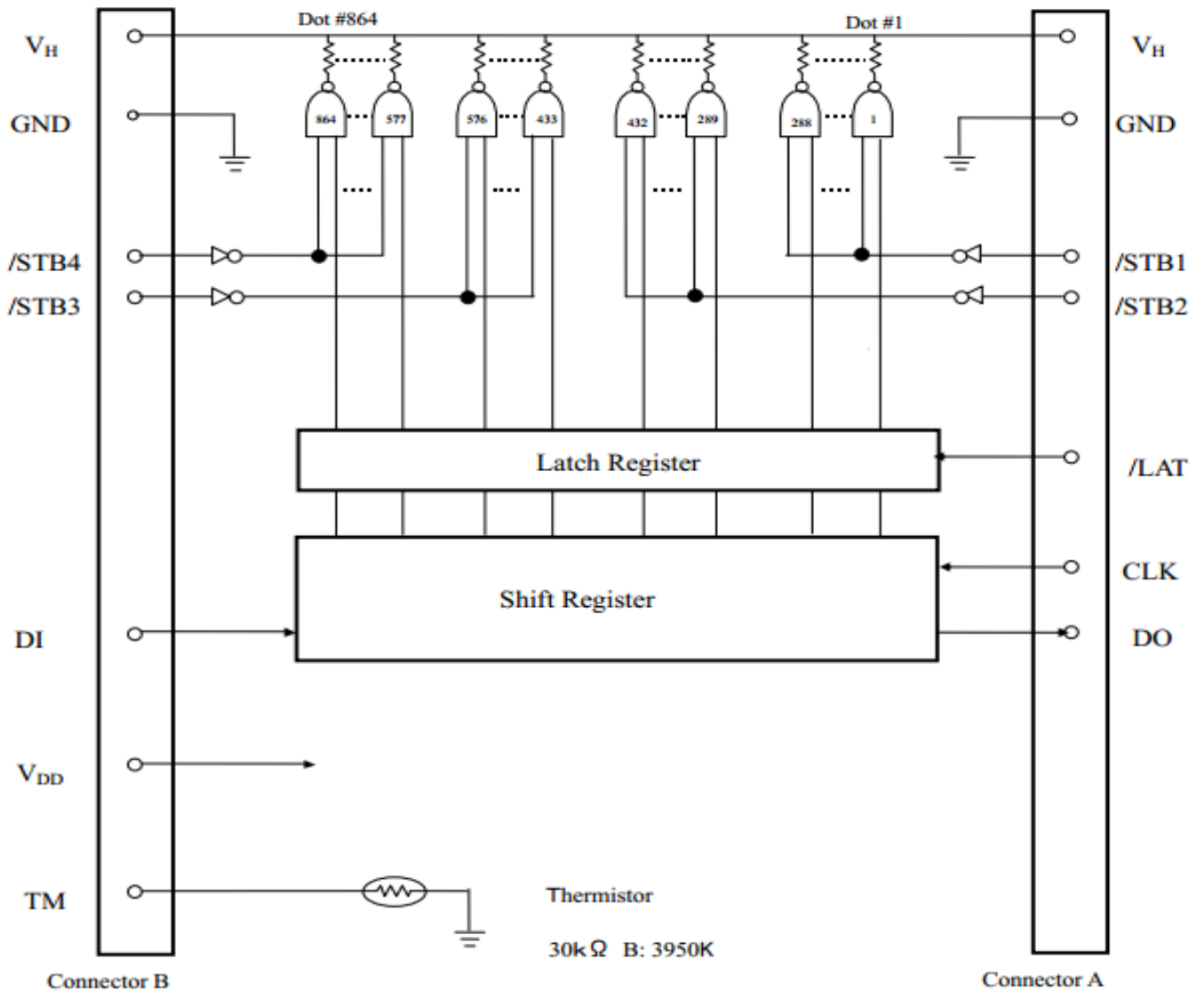
图 2 等价回路
