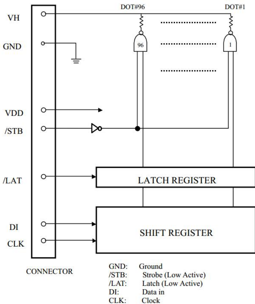
图 2 等价回路
