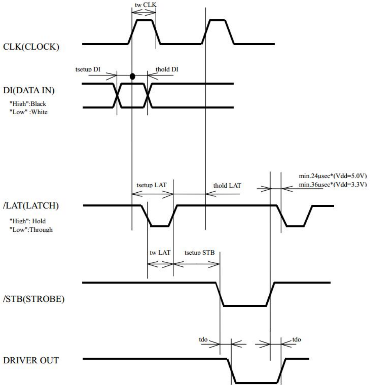
图 3 时序图
